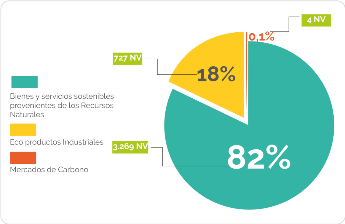
Gráfica 3 Participación de las categorías en el total de negocios verdes.
