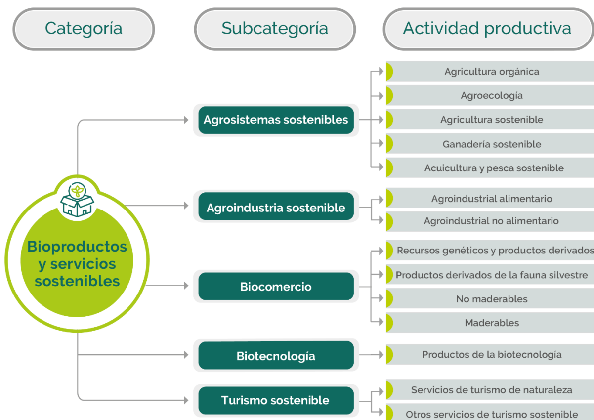
Ilustración 15 Clasificación de la categoría bioproductos y servicios sostenibles.
